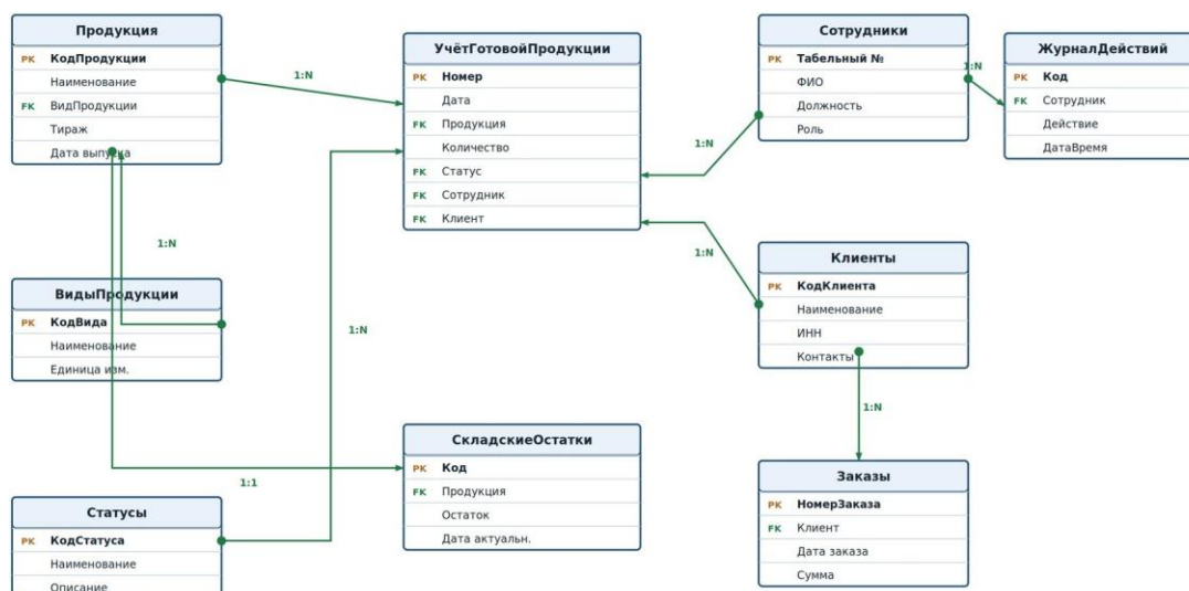
ER-диаграмма базы данных (логическая модель)
